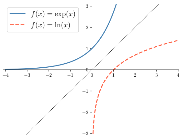
FIGURE 3.5 - Graphes des fonctions \exp et \ln .
