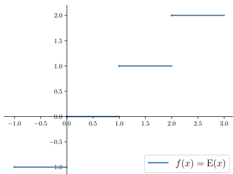
FIGURE 3.1 - Graphe de la fonction partie entière.
