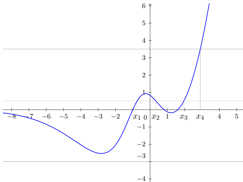
FIGURE 4 – Un exemple de fonction (non injective, non surjective)
