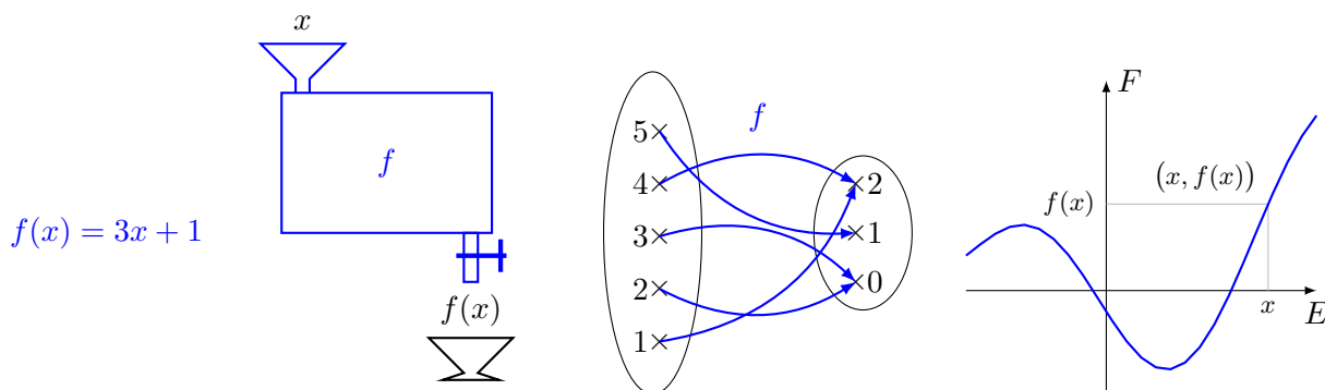
FIGURE 3 – Quatre images d’une fonction : (a) comme formule (insuffisant) ; (b) comme « machine » (très informel) ; (c) par un diagramme sagittal ; (d) par son graphe
