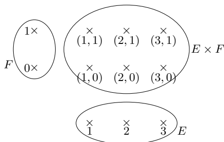
FIGURE 1 – Un exemple de produit cartésien : E = \{1, 2, 3\} , F = \{0, 1\}
