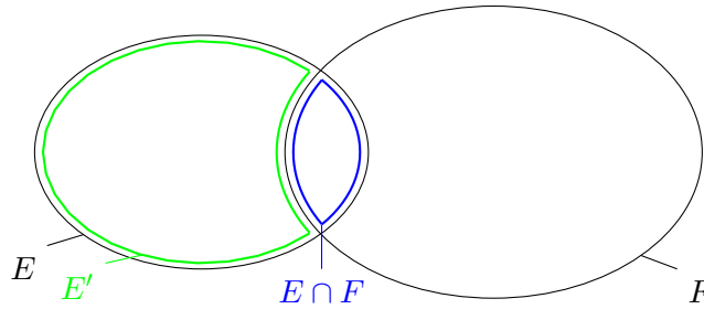
FIGURE 2 – Décomposition d'une réunion en parties disjointes
