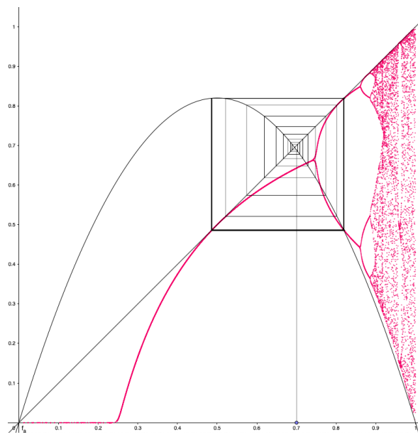
FIGURE 10.4 – Une suite u_{n+1} = f_a(u_n) pour a \approx 3,36 , et (en rouge) les points d'accumulation (\frac{a}{4}, u_n) pour n grands et différentes valeurs de a .
