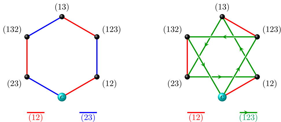
FIGURE 1.3 – Deux graphes de Cayley pour S_3 .
